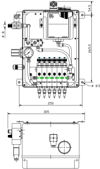
AFMETINGEN UCGF - SE
